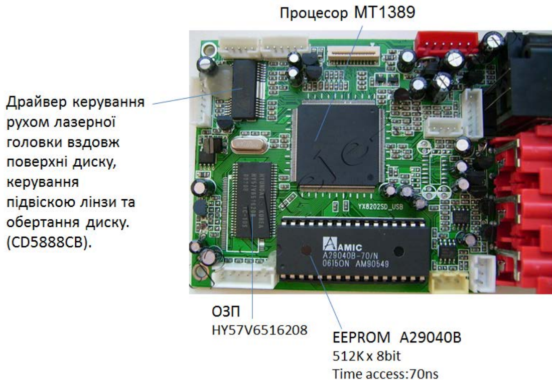
Рисунок 11 – Основна плата програвача CD/DVD
