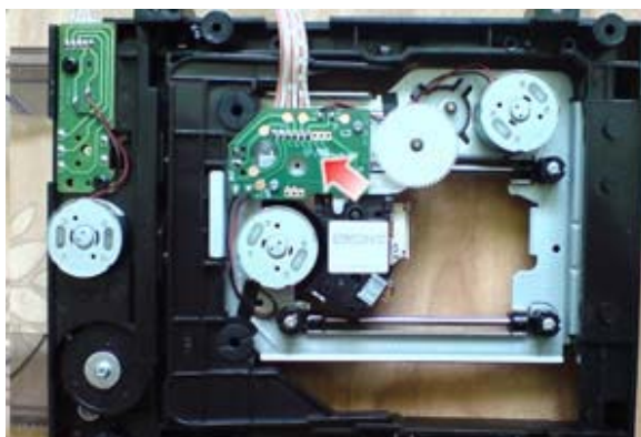
Рисунок 5 – Плата, на якій встановлений оптичний блок
