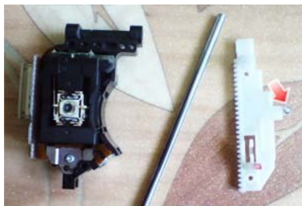
Рисунок 9 – Місце установки пружинки на зубчастій планці
