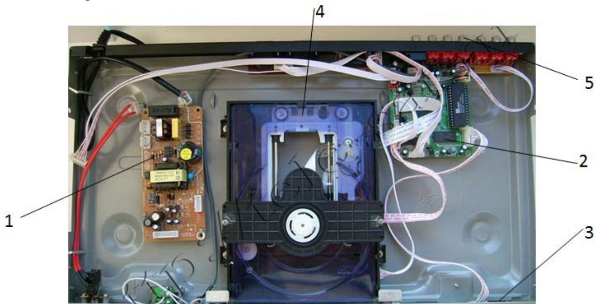
Рисунок 1 – Загальна конструкція програвача CD/DVD
