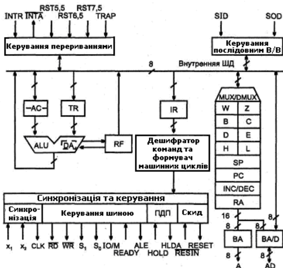
Рисунок 3 – Архітектура мікропроцесора K1821BM85A
